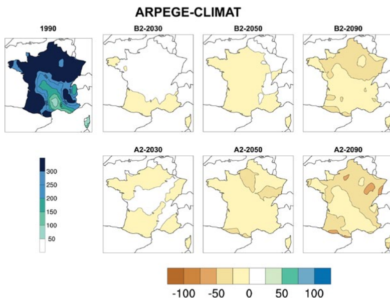
Figure H01-été. Minimum estival du contenu en eau du sol, pour la période de référence et les écarts entre les scénarios et la référence. Unité : kg/m 2 .
