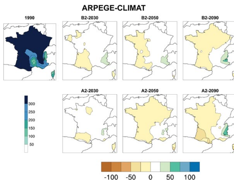
Figure H01-hiver. Minimum hivernal du contenu en eau du sol, pour la période de référence et les écarts entre les scénarios et la référence. Unité : kg/m 2 .
