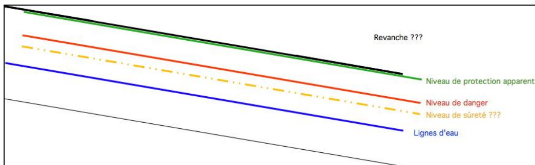
b- Digue en état imparfait et non munie d'un déversoir.
