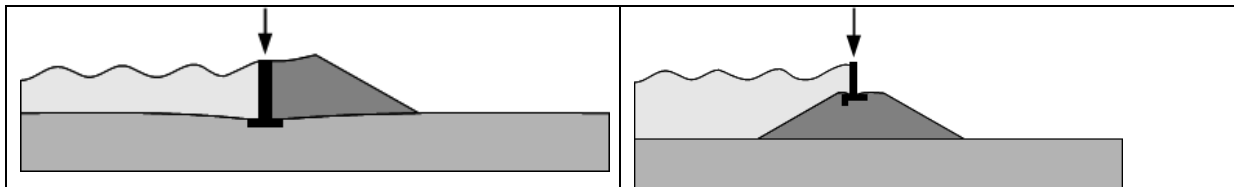
Figure 2.13 : Poinçonnement d'ouvrages rigides inclus dans une digue composite (Traduit et adapté de l'ILH)
