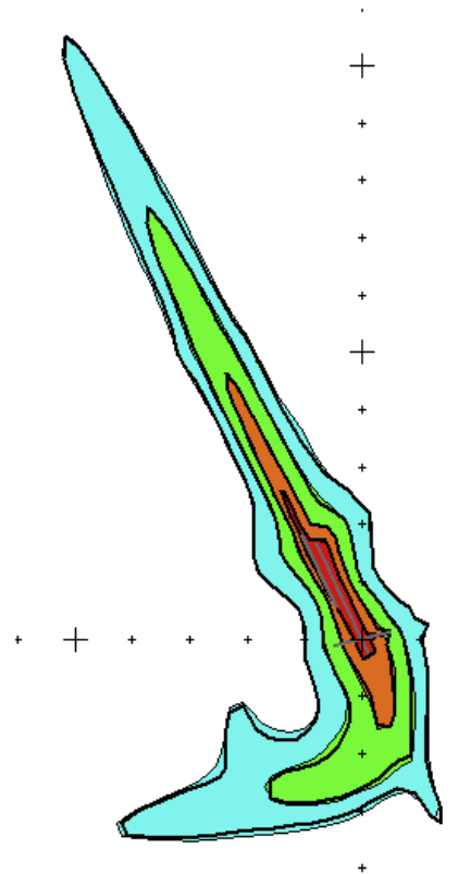
PEB avec INM 6.1 (sans DHC830)
